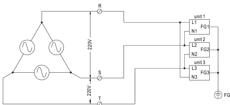
■ FIG. A: 3 \phi 3W 220VAC SYSTEM
